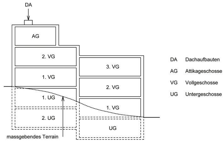
Geschosse und Geschosshöhe bei gestaffelten Gebäuden
